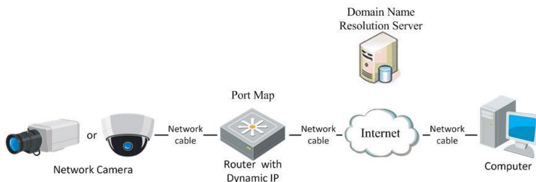
Figure 2-13 Zuweisung eines privaten Domain-Namens
