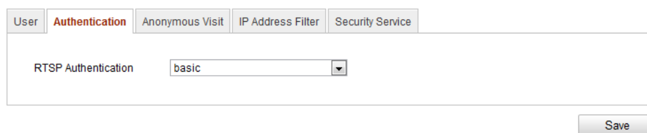
Figure 12-4 RTSP-Authentifizierung
