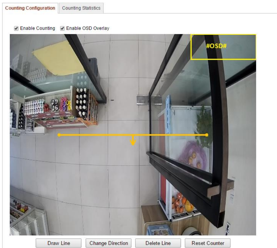
Figure 8-1 Zählungskonfiguration
