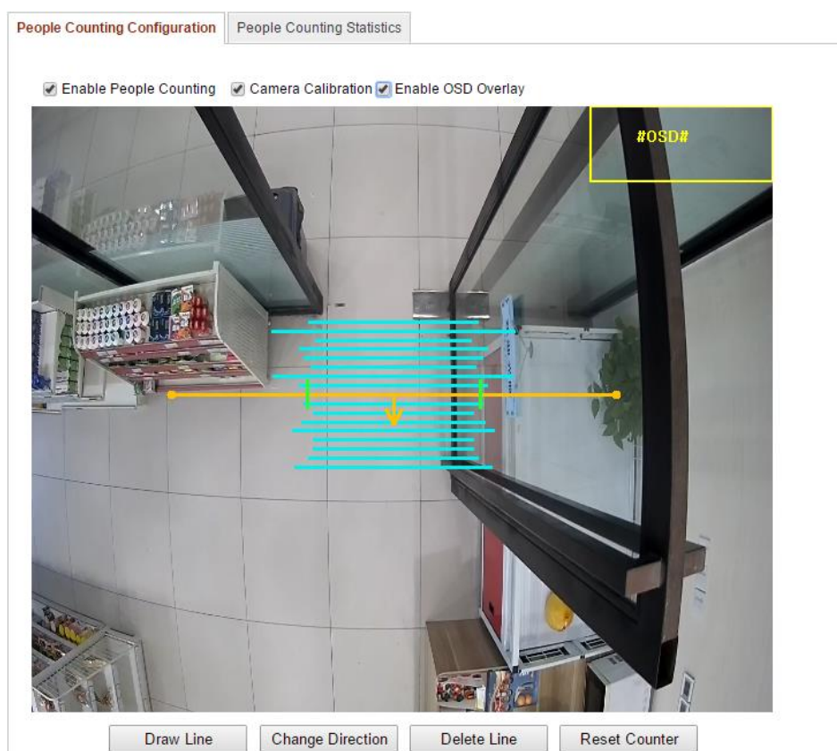
Figure 6-76 Personenzählung-Konfiguration
