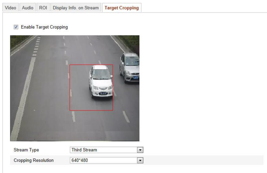
Figure 6-33 Zielfreistellung
