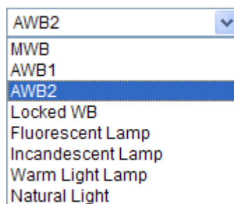
Figure 6-36 Weißabgleich
