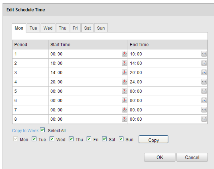
Figure 6-46 Aktivierungszeitplan
