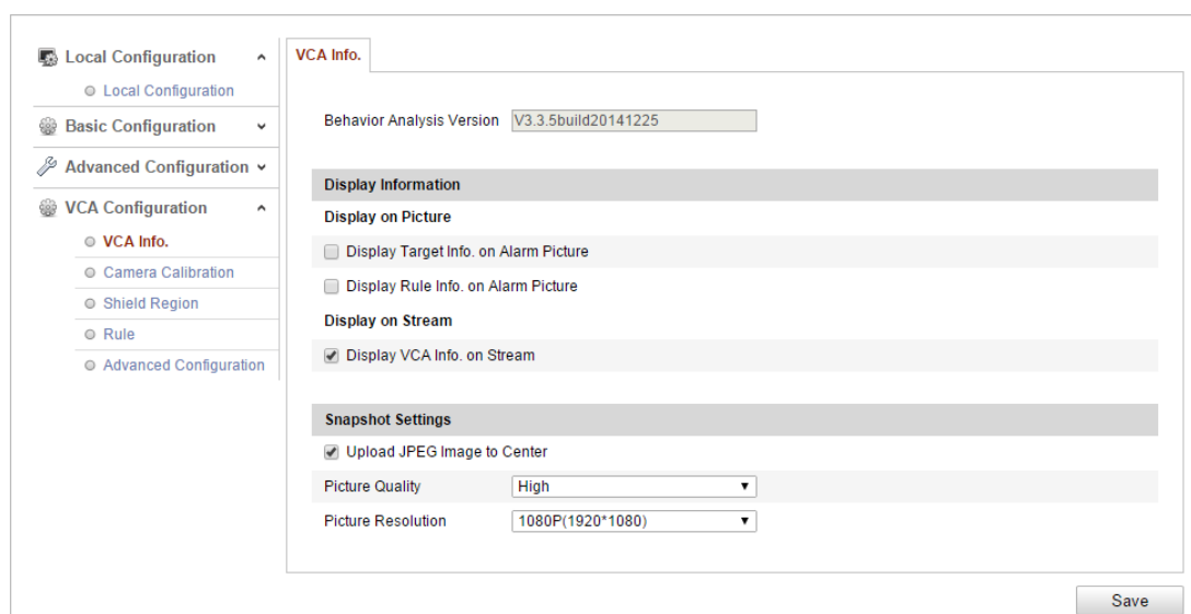
Figure 6-68 Verhaltensanalyse
