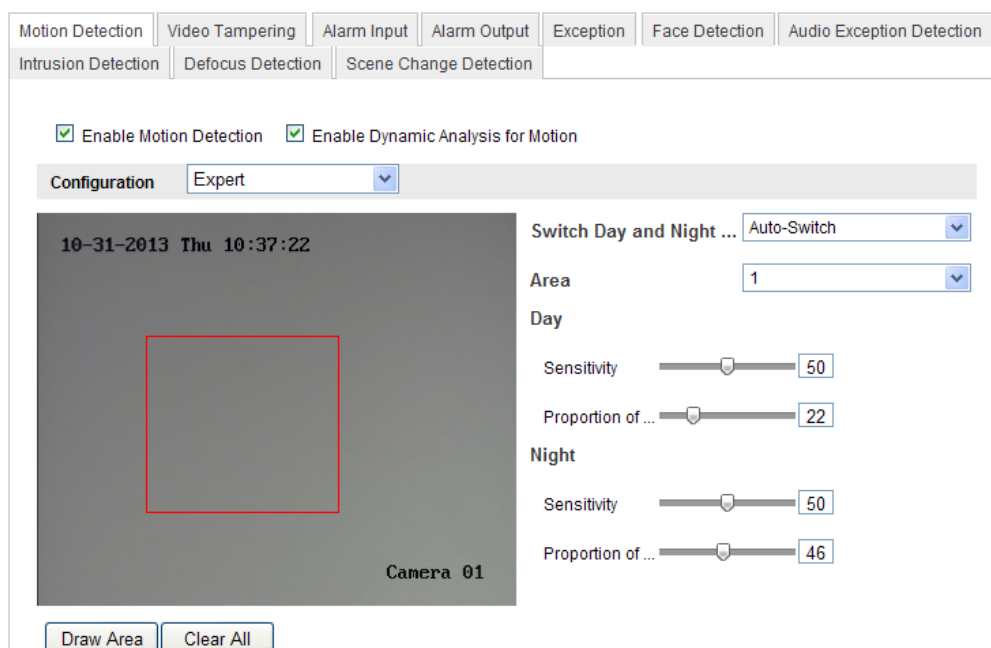
Figure 6-49 Automatische Tag/Nacht-Umschaltung
