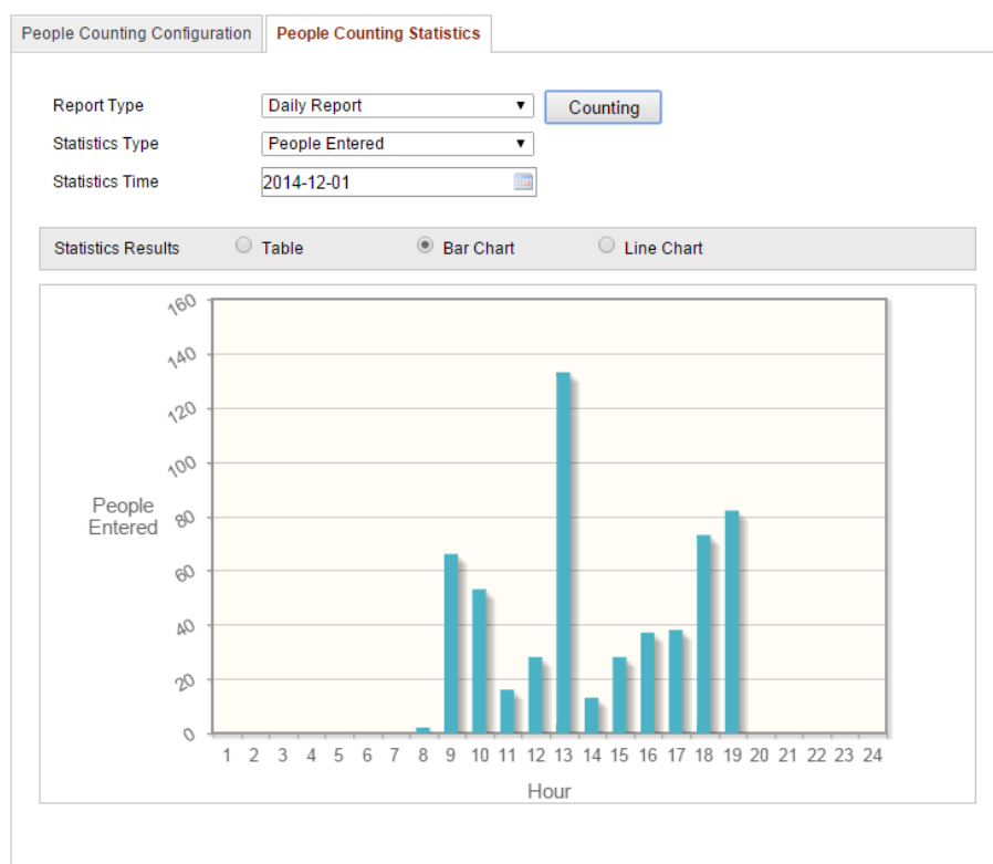
Figure 6-77 Statistikergebnisse
