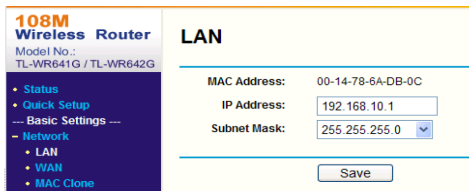
Abbildung A.2.2 – Konfigurieren der LAN-Parameter
