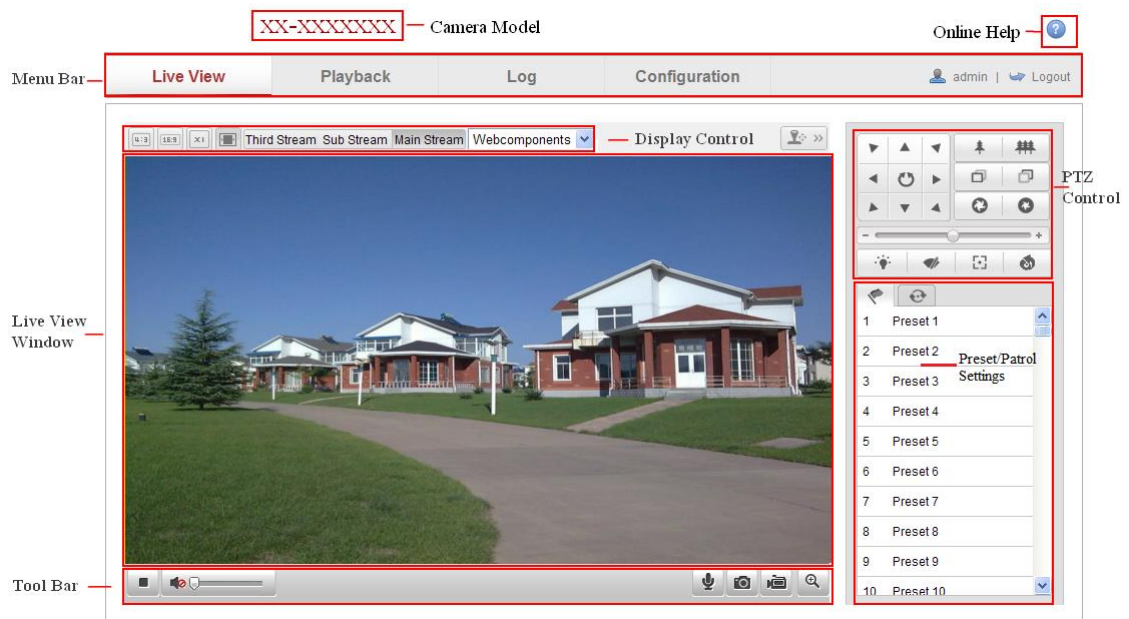
Figure 5-1 Liveansicht-Seite
