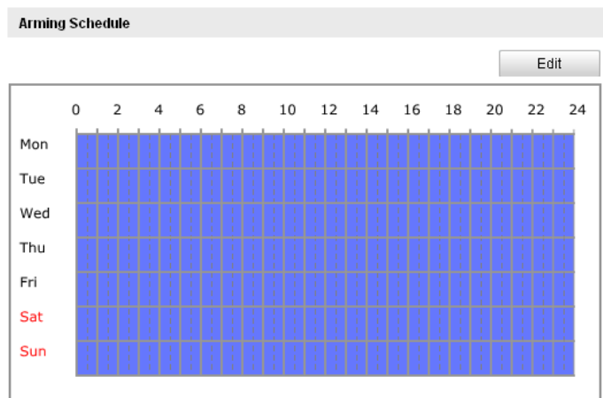
Figure 6-45 Aktivierungszeit
