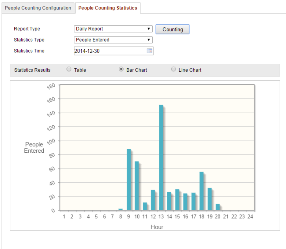
Figure 8-2 Statistikergebnisse
