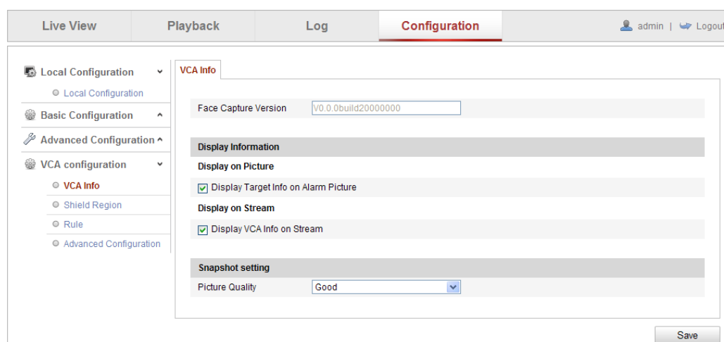
Figure 6-72 Gesichtserfassung
