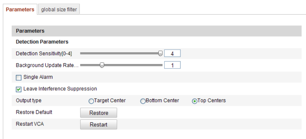
Figure 6-71 Weiterf. Konfiguration
