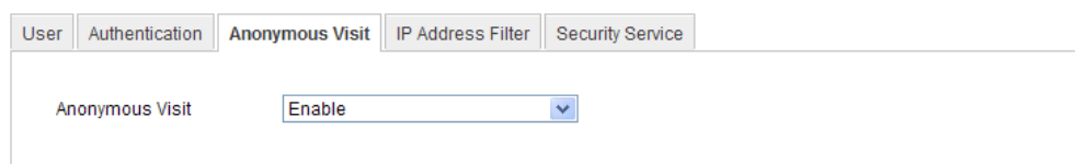
Figure 12-5 Anonymer Besuch
