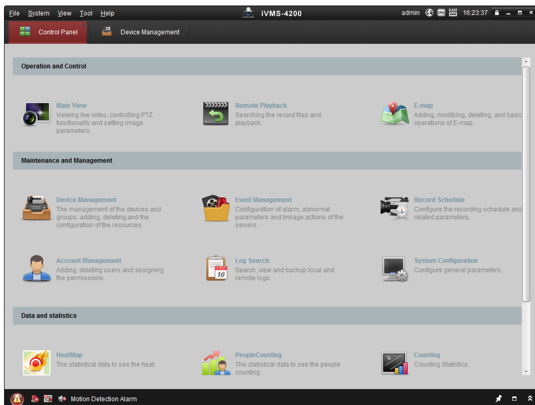
Figure 3-5 iVMS-4200 Systemsteuerung
