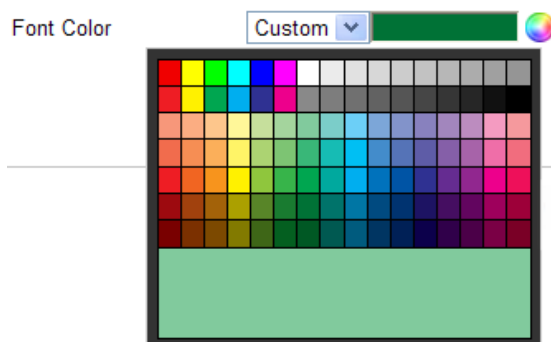
Figure 6-39 Schriftfarbe – Benutzerdefiniert
