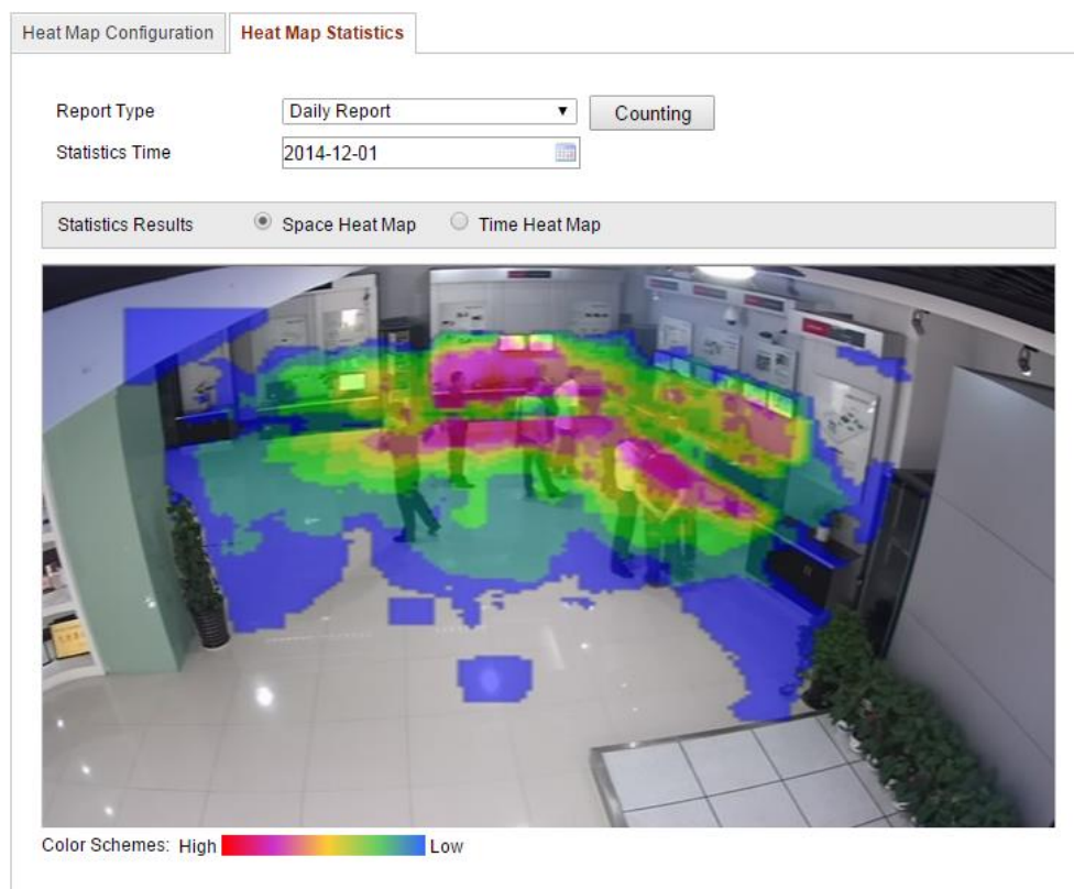
Figure 6-75 Platz-Wärmekarte
