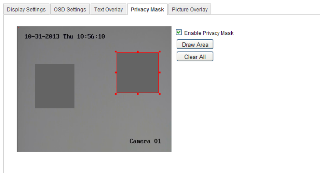
Figure 6-42 Privatzonen-Maskierungseinstellungen
