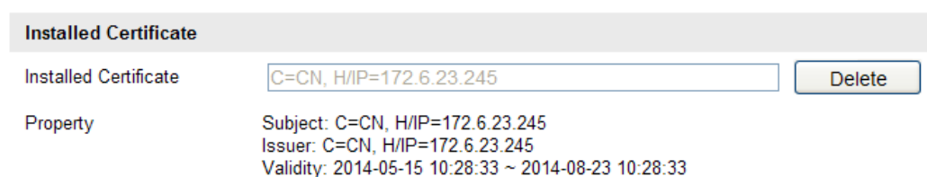
Figure 6-28 Installiertes Zertifikat
