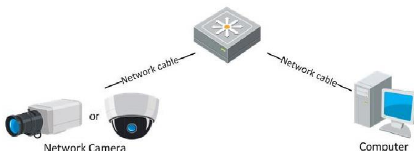
Figure 2-2 Anschluss via Switch oder Router
